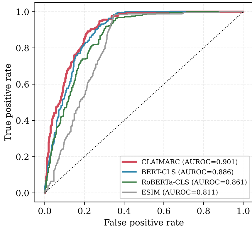
(b) ROC
