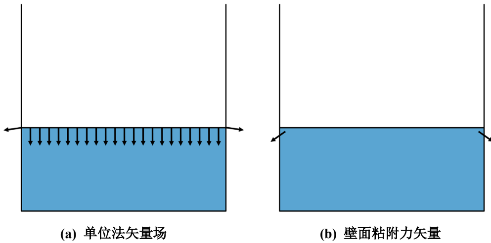
图 4.13 CSF 算例的初始单位法矢量场和壁面粘附力矢量
