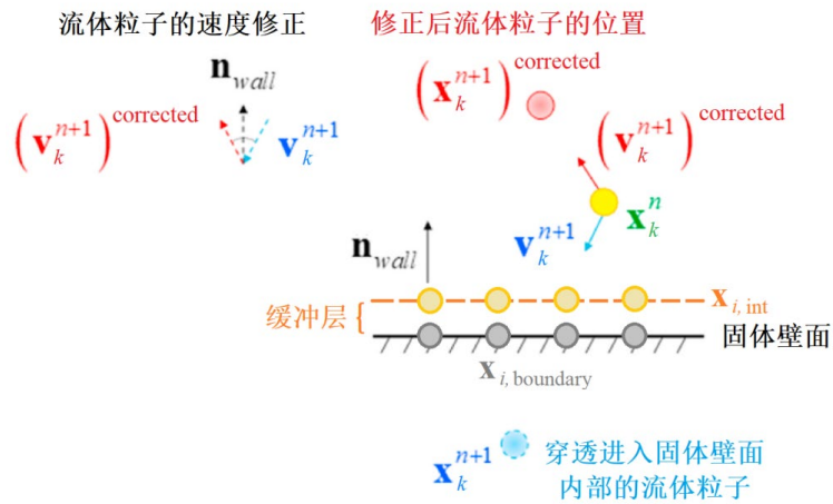
图 4.3 固体壁面的碰撞模型
