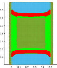
inpolygon
