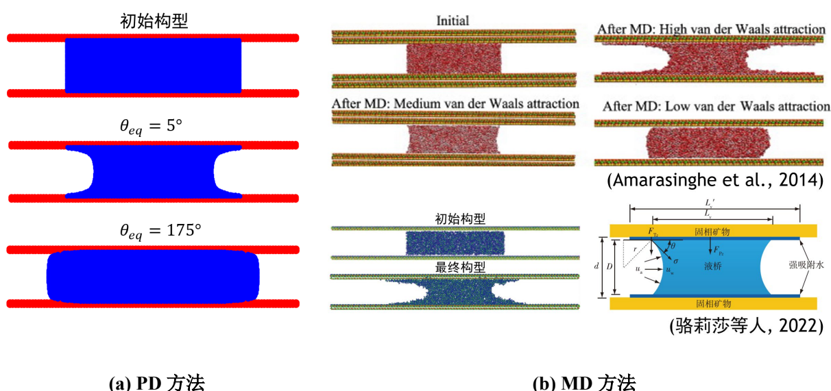
图 14 不同算例的弯液面最终形态
