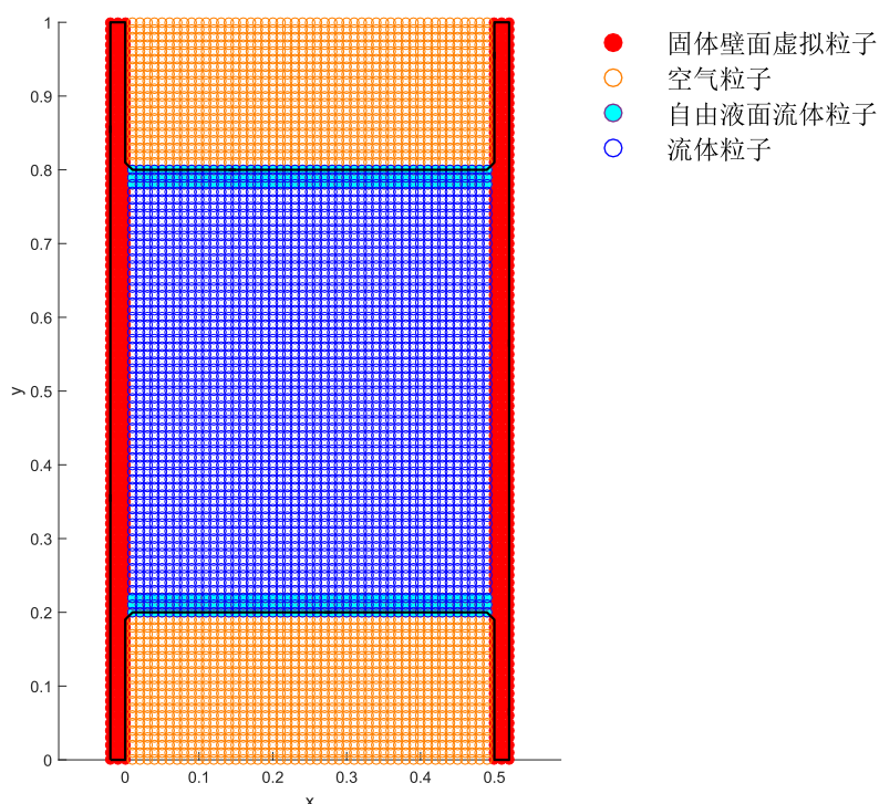
图 2 单液桥模型的几何示意图
