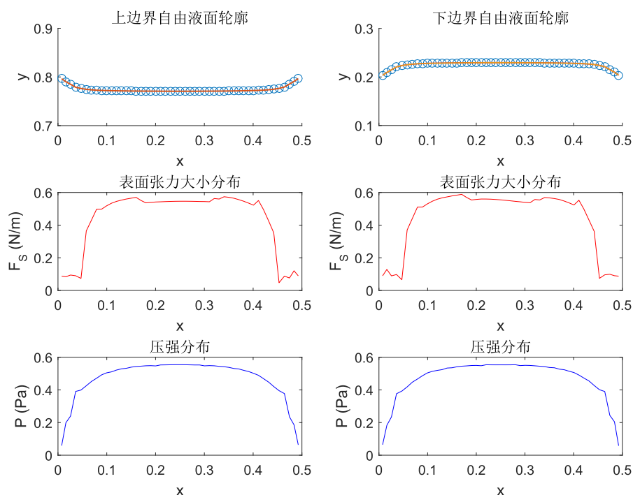
图 13 凹液面表层粒子的表面张力分布和压强分布
