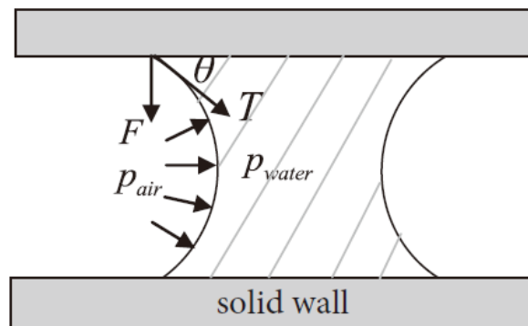
图 1 单液桥模型
