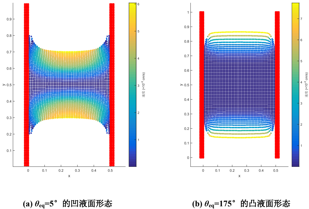
图 10 最终构型粒子速度大小分布
