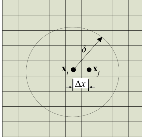
图 4 二维结构的中心正交均匀离散
