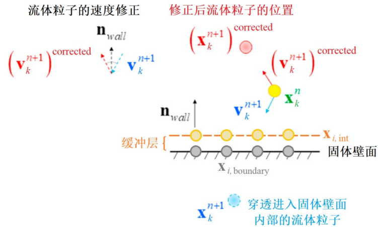
图 6 固体壁面的碰撞模型
