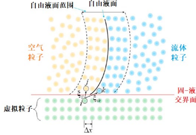
图 5 固体壁面边界处理
