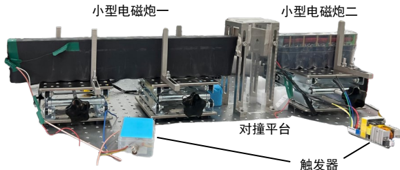
小球对撞实验台
