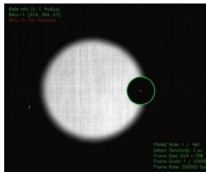
两小球碰撞瞬间(20万帧)
