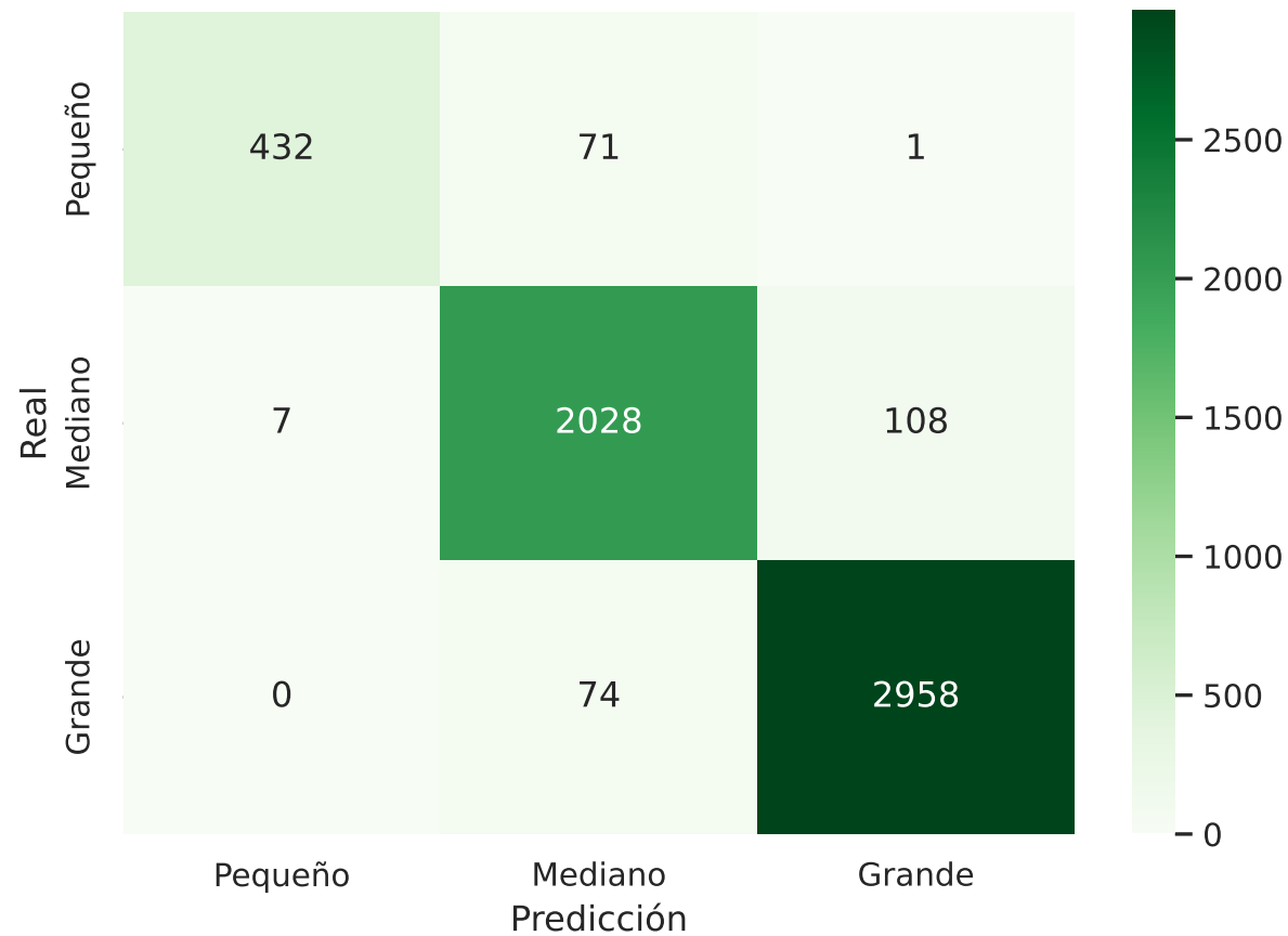
Random Forest — Matriz de Confusión Tamaño
