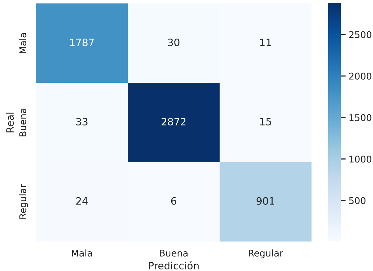
Random Forest — Matriz de Confusión Calidad
