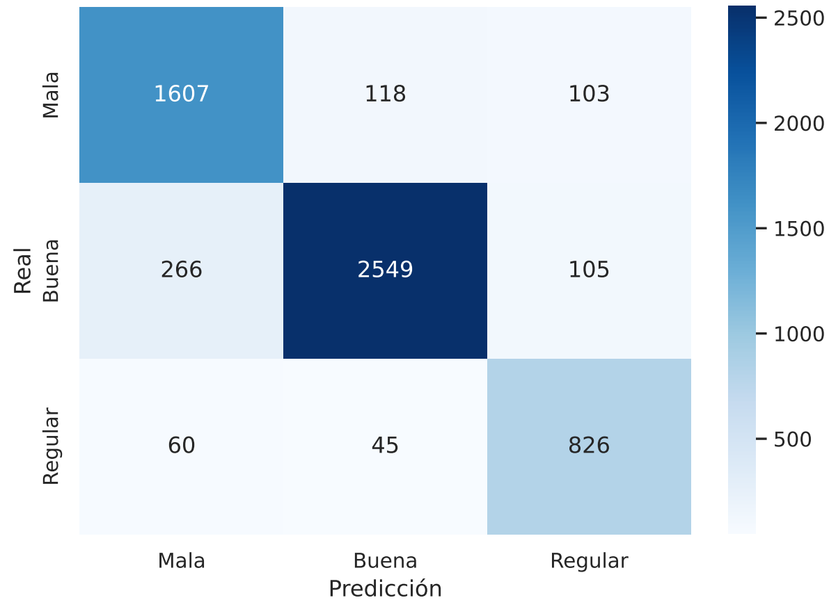
SVM lineal — Matriz de Confusión Calidad
