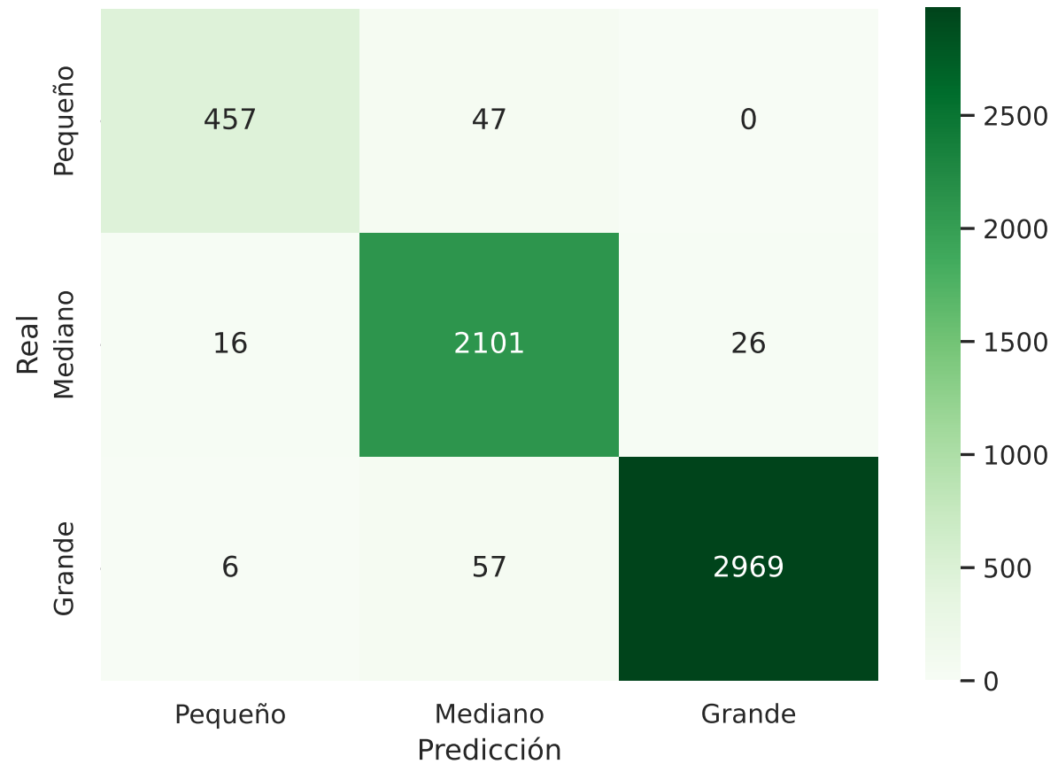
SVM lineal — Matriz de Confusión Tamaño
