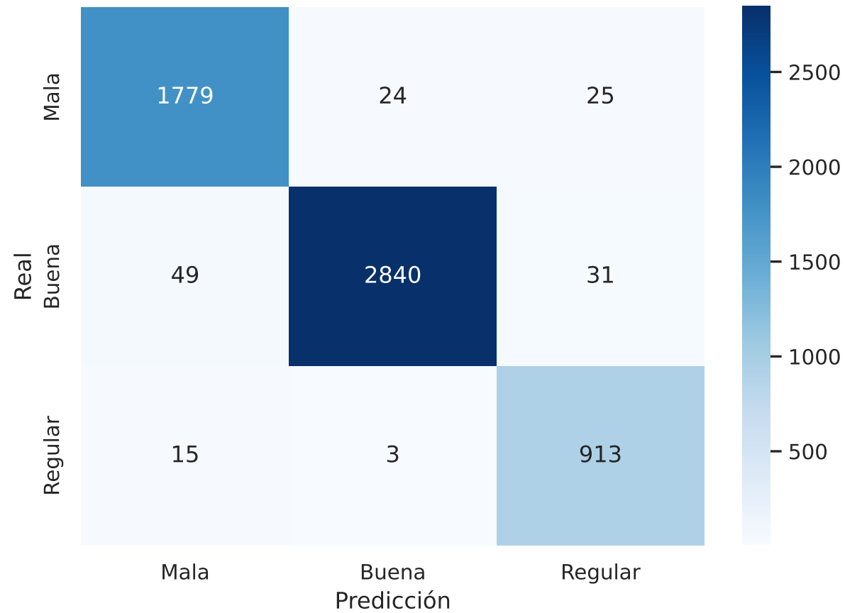
XGBoost — Matriz de Confusión Calidad
