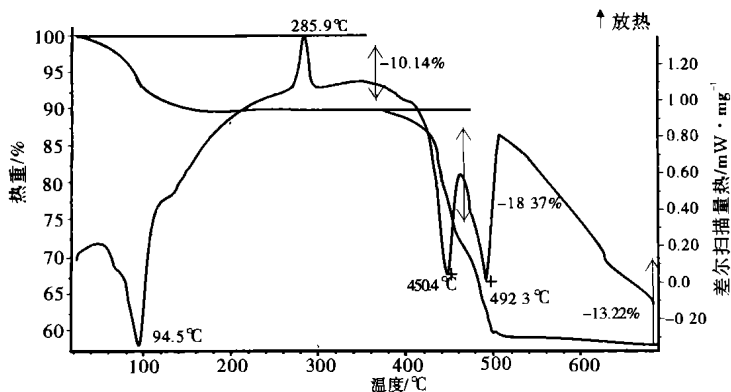
2. \text{K}_3[\text{Cr}(\text{C}_2\text{O}_4)_2] \cdot 3\text{H}_2\text{O}
