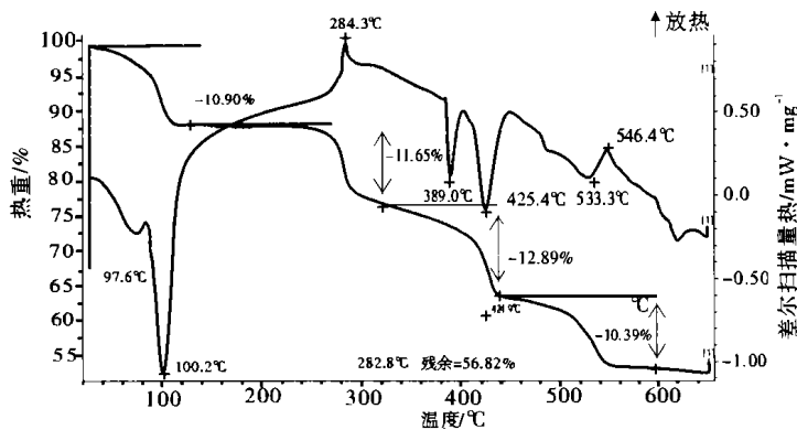
3. \text{K}_3[\text{Fe}(\text{C}_2\text{O}_4)_3] \cdot 3\text{H}_2\text{O}
