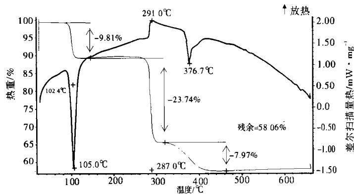
4. K_3[ Cu(C_2O_4)_2 ] \cdot 2H_2O
