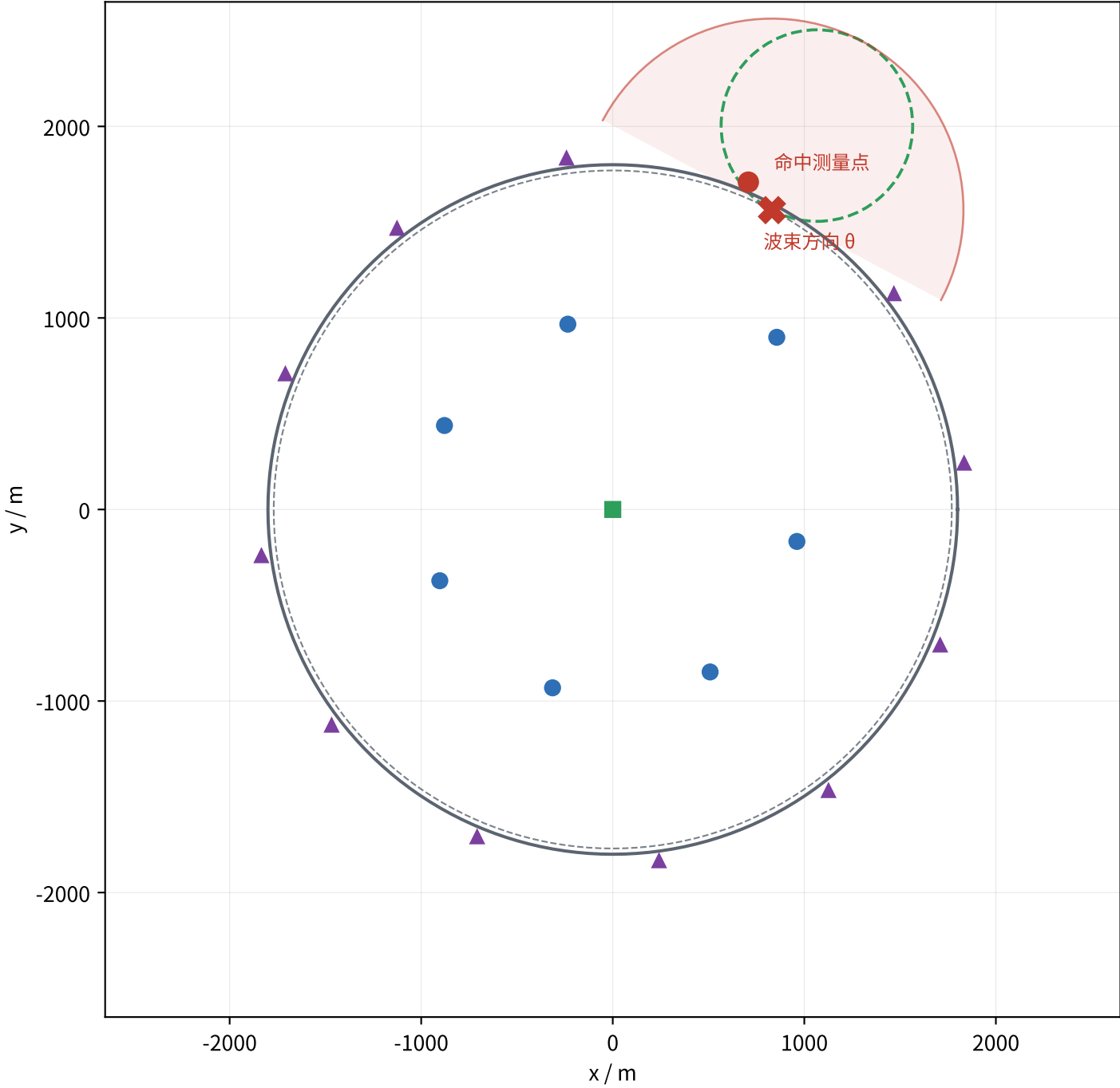
扫描布局：原点 + 7 覆盖基点 + 12 均匀外圈点（20 个测量位置，里程 17.00 km，实测听到率 99.9891%）
