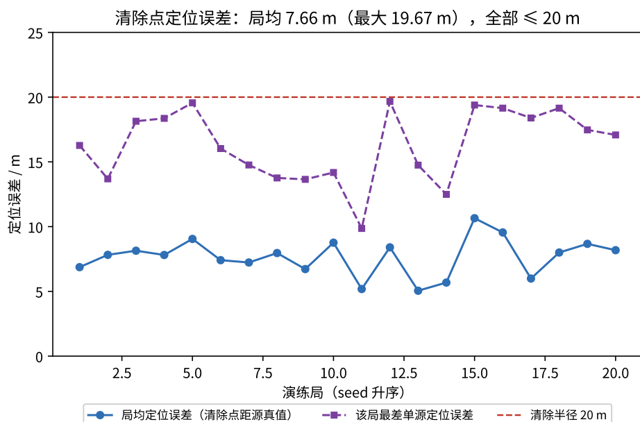
图 5: 清除点定位误差：局均 7.66 m，全部落在 20 m 清除半径内。
