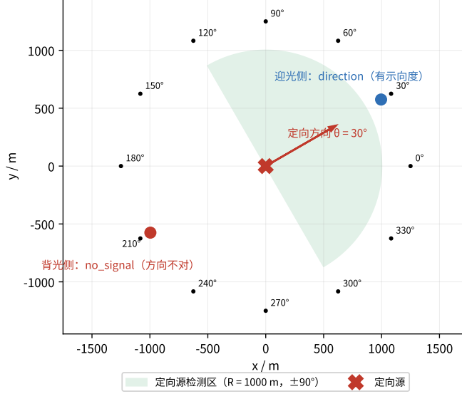
图 1: 定向源”方向不对”示意：波束迎光侧返回 direction，背光侧返回 no_signal，机器狗必须走到源正面才能听到。
