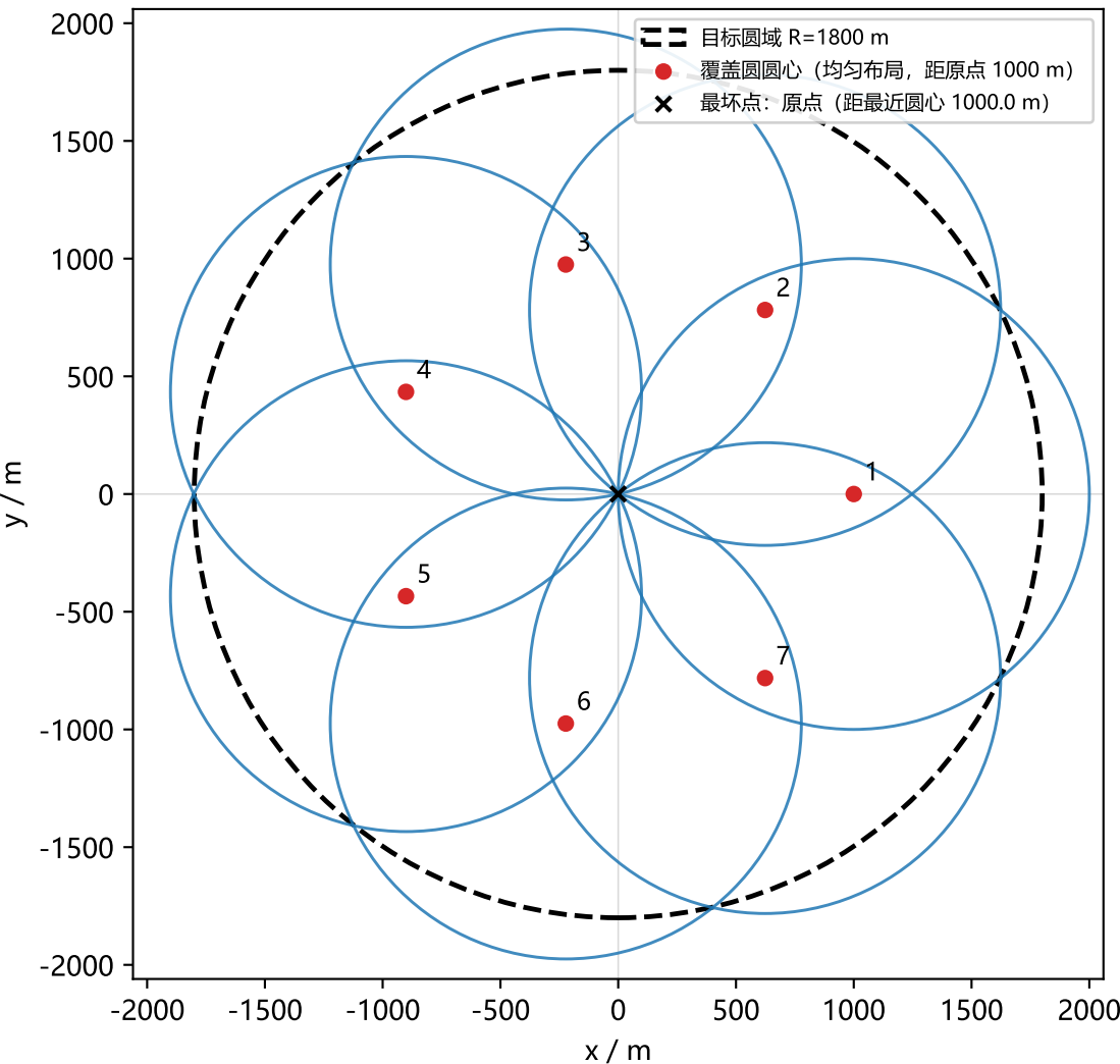
7 个半径 1000 m 覆盖圆 (均匀布局) 覆盖半径 1800 m 圆域
