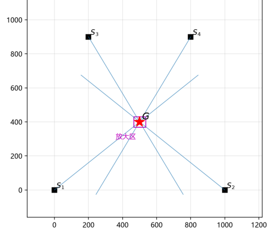
图 2: 四个检测点的交会布局
