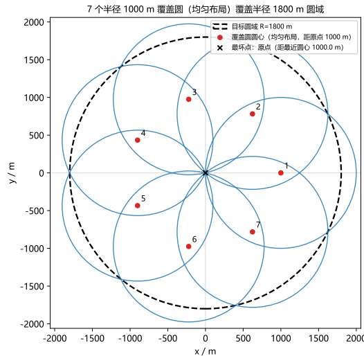
图 8: 均匀布局: 7 个半径为 1000 m 的覆盖圆覆盖半径 1800 m 的目标圆域
