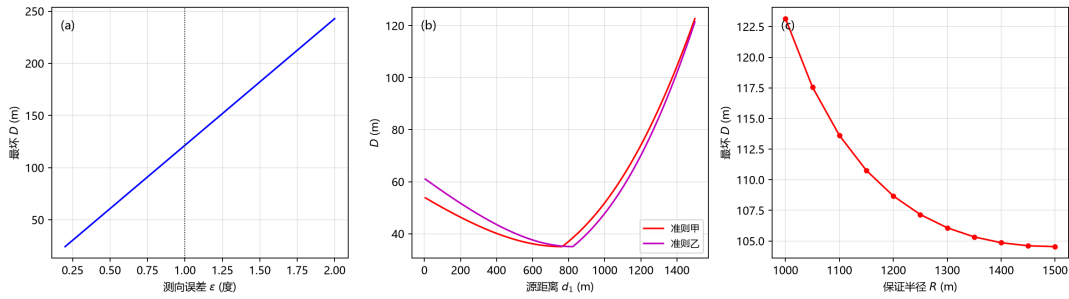
图 7: (a) D 对 \varepsilon (b) D 随 d_1 (c) 最坏 D 对保证半径 R 。
