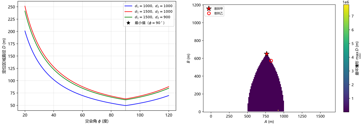
(a) 定位区直径 D 随交会角 \phi 的变化
