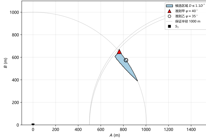
图 6: 第二检测点候选区域与两条准则的推荐落点。
