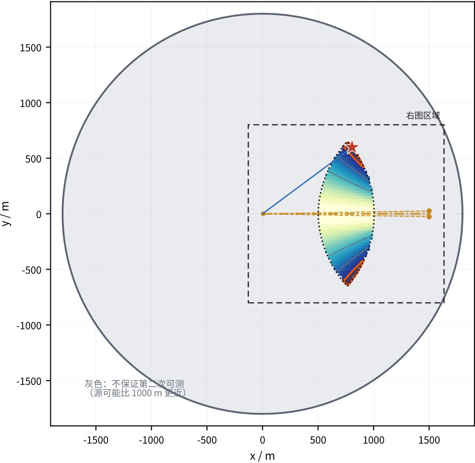
(a) 全域：1800 m 圆域、源不确定集与适合度
