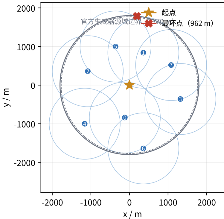
覆盖路点布局 (8 个, 半径 920 m)
