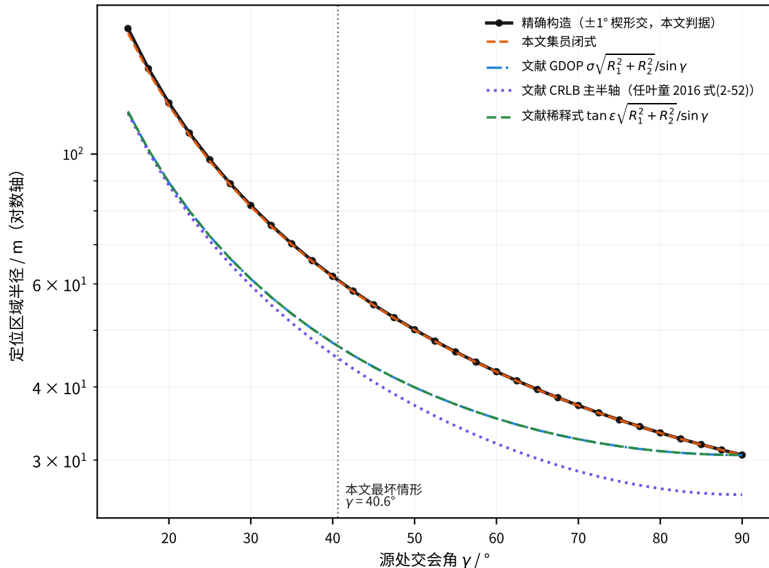
(a) 交会角的影响 ( R_1 = 1500 m, R_2 = 907 m)
