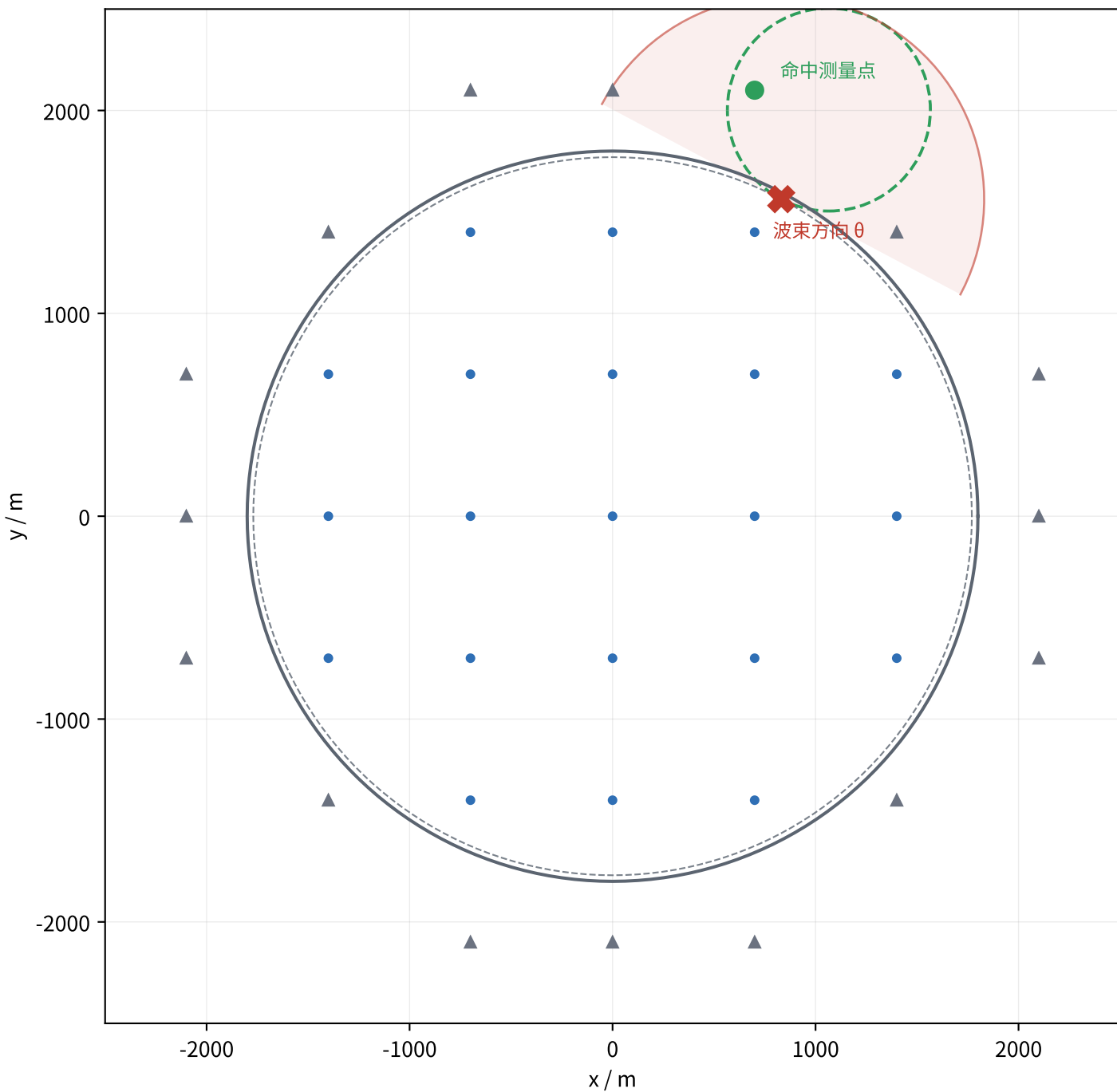
寻向拖网：间距 700 m 格点取到半径 2270 m (37 个测量点，保证命中任意半圆盘)
