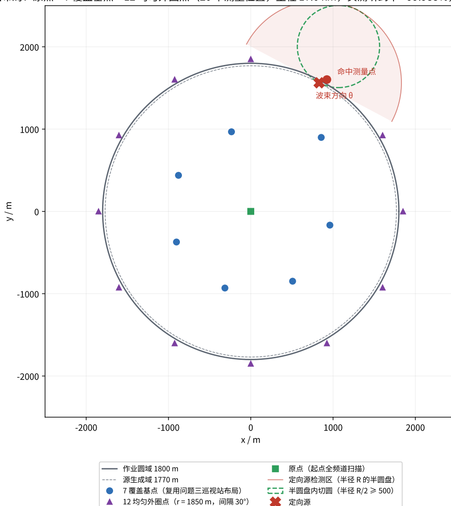
图 2: 检测扫描布局 (20 点定案): 原点 + 7 覆盖基点 + 12 均匀外圈点; 红色半圆盘为某贴边定向源的检测区示意 (半径 R = 1000 m、波束朝外), 其内切圆内必有测量点命中。
