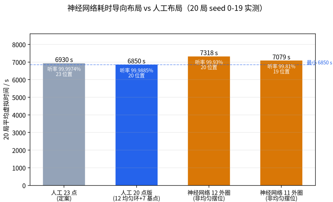
图 8: 各布局 20 局实测平均虚拟时间：人工 20 点版 6850 s 为最小，神经网络全部尝试（自由、12 外圈、11 外圈）均更慢。
