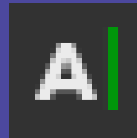
Herramienta Texto
