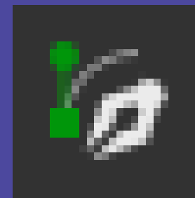
Herramienta Pluma
