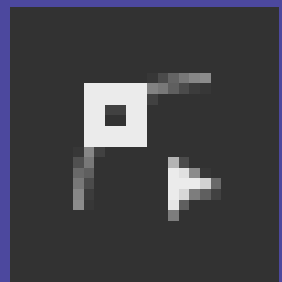
Herramienta nodo
