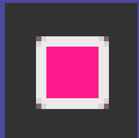
Herramienta Rectángulo
