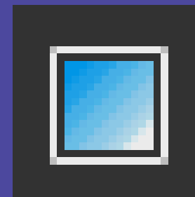
Herramienta Degradado
