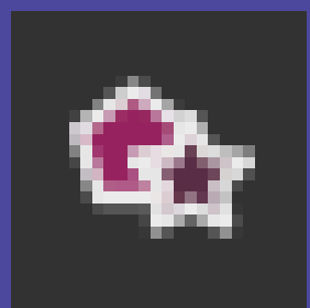
Herramienta Estrella/Polígono
