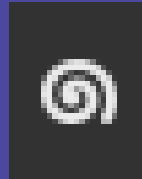
Herramienta Espiral
