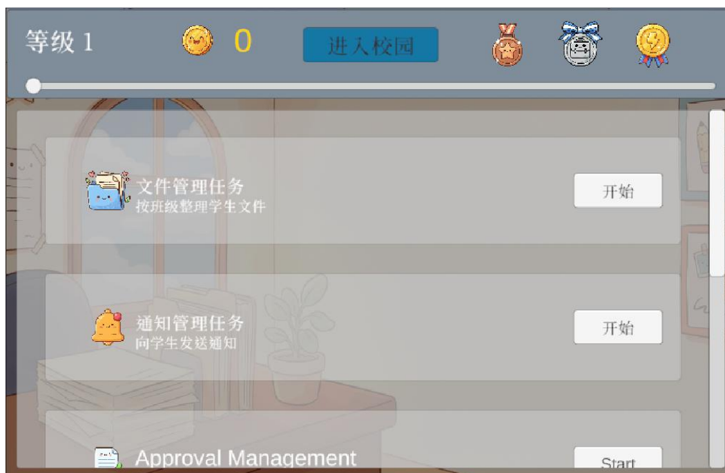
图 2：主菜单界面
