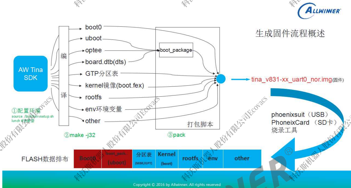
图 4-2: SDK 整体数据流程
