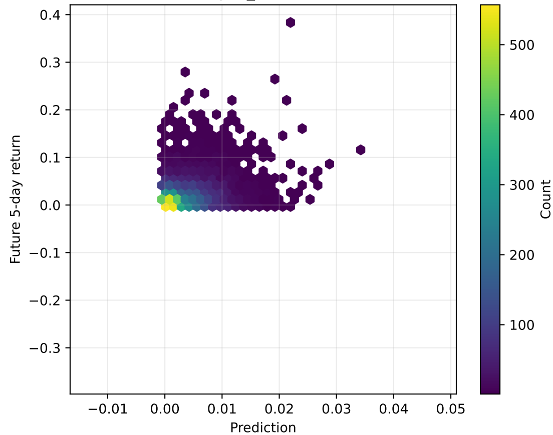
hcgnn_continual
