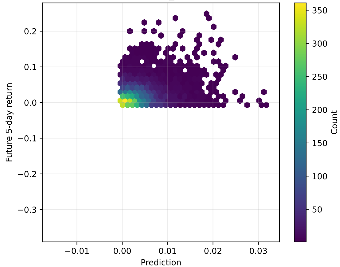
protocol_gnn
