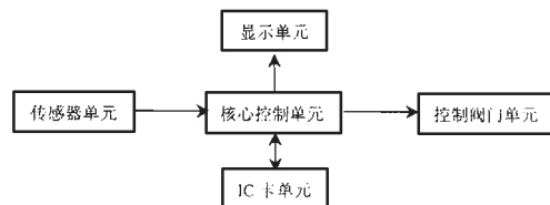
图 1 IC 卡水表系统的基本结构框图
