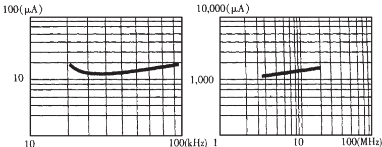
图 3 87LPC764 工作电流与频率关系
