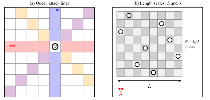
图 1. (a) 一个皇后 (黑色圆圈) 及其在 8 \times 8 棋盘上的四条攻击线: 行 (红色)、列 (蓝色)、主对角线 (橙色)、反对角线 (紫色)。 (b) Q(8) = 92 个非攻击构型之一, M = N = 8 个皇后。在理想气体类比中 (第 III 节), 物理棋盘边长 L = N\lambda 扮演容器尺寸的角色, 其中 \lambda (一个格点宽度) 是类似于热 de Broglie 波长的格点间距, \ln(L/\lambda) = \ln N 给出单粒子”相空间”熵。
