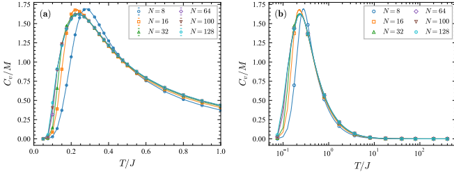
图 3. M = N 时每个皇后的比热 C_v/M 与 T 的关系。(a) 峰值区域 ( T \leq 1 J , 线性标度), 附误差棒。(b) 对数 T 标度下的全温度范围。 M \geq 32 的曲线坍缩到单一函数上, 确认了向热力学极限的收敛。
