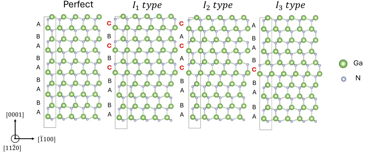
圖 3.2：氮化鎵晶體堆疊錯誤類型 [PhysRevB.71.235334, liliental2014structural, komninou2005partial]。
