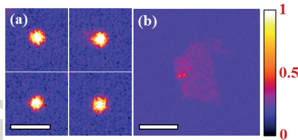
圖 1.2：(a) 缺陷 h-BN 的 SHG 強度圖，明顯高於無缺陷結構。(b) 因經由機械剝離的 h-BN 其缺陷較少，圖中也可觀察到其 SHG 強度較微弱。[Cunha_2020]
