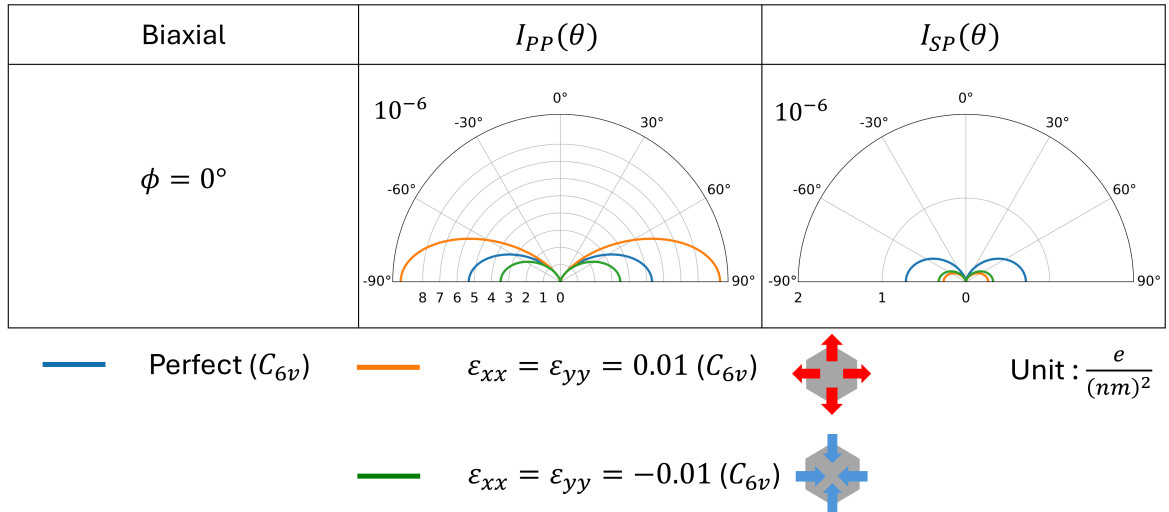
圖 3.14：當 \phi = 0^\circ ，入射光與出射光皆在 xz 平面，雙軸應變結構與於缺陷結構的 SHG 強度與 \theta 角度的關係比較。
