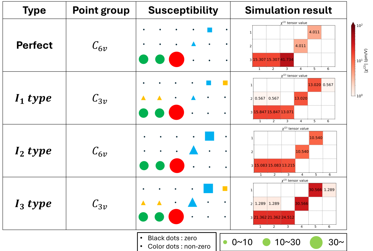
圖 3.3：氮化鎵不同的堆疊錯誤缺陷類型的 SHG 模擬結果。極化率張量一欄是將模擬結果一欄的數值簡化表示：正方形表示為會影響 P_x 分量；三角形表示為會影響 P_y 分量；圓形表示為會影響 P_z 分量；黑色的小點表示其值為零。顏色相同表示其絕對值相同。在表格最後一欄為第一原理模擬出的極化率張量 \chi^{(2)} 的絕對值。我們選擇能量為 1.181eV(波長為 1050nm) 作為分析標準，取該能量下的極化率張量分量值進行比較與討論。
