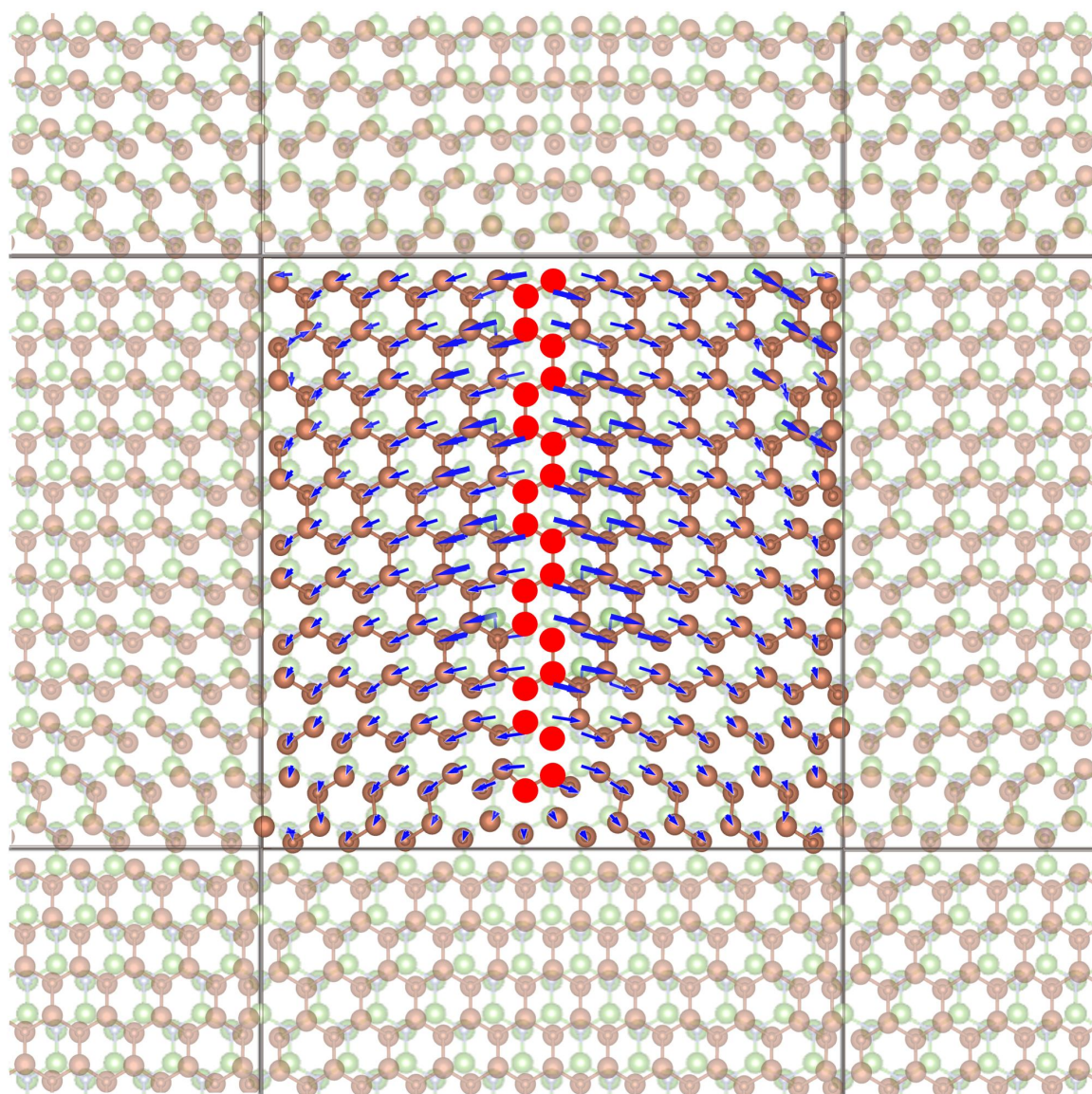
圖 3.4：刃狀差排結構相對無缺陷結構的原子位移圖。利用 AtomsK 軟體 [hirel2015atomsK] 設定刃狀差排的差排線 (Dislocation line)[0001]，以及伯格斯向量 (Burgers vector)[11 \bar{2} 0] 生成 GaN 的刃狀差排結構。綠色透明的部分為完美的 GaN 結構；深紅色為含有刃狀差排的結構；紅色圓圈標示刃狀差排的位置；藍色箭頭為表示超晶胞中的原子因刃狀差排的插入而被向外推擠，產生的位移，箭頭方向表示位移方向，箭頭長度表示位移的大小。
