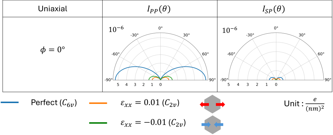
圖 3.13：當 \phi = 0^\circ ，入射光與出射光皆在 xz 平面，單軸應變結構與於缺陷結構的 SHG 強度與 \theta 角度的關係比較。
