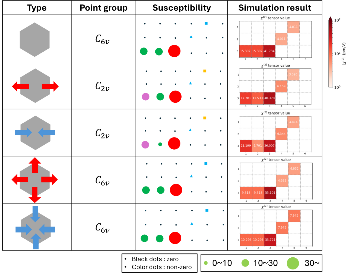
圖 3.7：對氮化鎵晶體作單軸應變，並模擬其二階極化率張量值。極化率張量一欄是將模擬解果一欄的數值簡化表示：正方形表示為會影響 P_x 分量；三角形表示為會影響 P_y 分量；圓形表示為會影響 P_z 分量；黑色的小點表示其值為零。顏色相同表示其絕對值相同。在表格最後一欄為第一原理模擬出的極化率張量 \chi^{(2)} 的絕對值。
