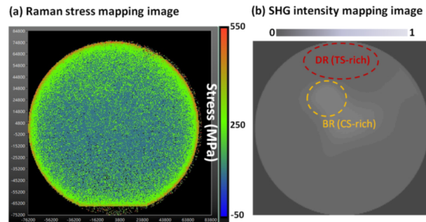
圖 1.1：(a) 透過拉曼光譜量測繪製出的應力分布圖。(b) 與 (a) 對應區域的 SHG 強度分布圖。[Chiang_2023]
