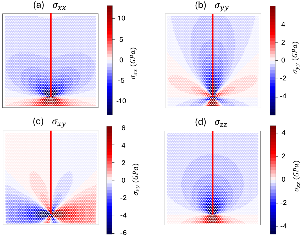
圖 3.5：使用 atomsk 軟體 [hirel2015atomsk] 將刃狀差排插入完美的晶格中，並可用解析的應力公式計算出應力的分布。紅色矩形標示的位置為刃狀差排。(a) 為 \sigma_{xx} ；(b) 為 \sigma_{yy} ；(c) 為 \sigma_{xy} ；(d) 為 \sigma_{zz} 。
