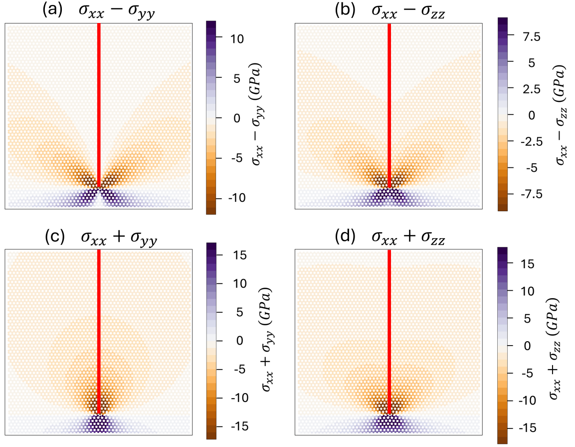
圖 3.6：(a) 為 \sigma_{xx} - \sigma_{yy} 。顯示在 x 方向與 y 方向應力相減後的分布，可以觀察到整體應力值變化不大，顯示主要貢獻來自 x 方向的應力。(c) 為 \sigma_{xx} + \sigma_{yy} 對應於圖 (3.5)(a) 與 (b) 的疊加結果，可見數值有所增加，但主要貢獻仍為 x 方向，而在差排附近，其數值大致落在 0 至 -5 的範圍內。(b) 為 \sigma_{xx} - \sigma_{zz} ，與圖 (3.5) 中的 (a) 與 (d) 相比，可以看出應力仍主要集中在 x 方向。(d) 顯示 \sigma_{xx} + \sigma_{zz} ，其數值確實進一步增加，但主要貢獻還是在 x 方向。綜合比較可知，刃狀差排在空間中主要引發的應力方向為 x 方向，並且在差排插入附近的區域會形成壓應力 (Compressive stress)。
