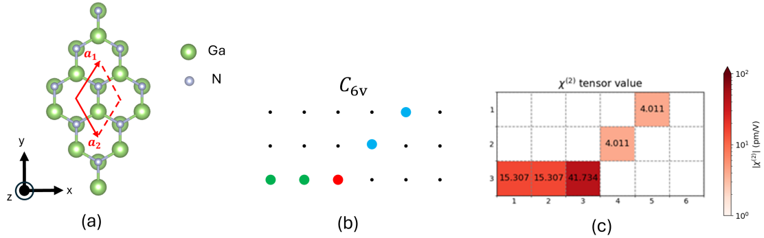
圖 3.1：(a) 無缺陷的 GaN 以及在 xy 平面上的晶格向量。(b) 為 C_{6v} 點群由 Neumann principle 推導出的二階極化率非零張量分布。黑色小點為零；有顏色的圓形為非零，顏色相同為值相同。(c) 為經 Abinit 軟體模擬出的二階極化率張量絕對值。
