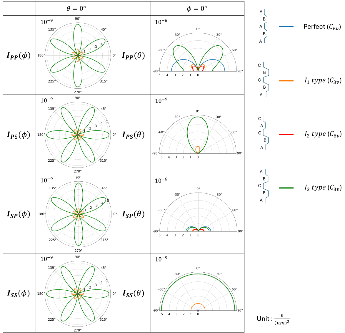
圖 3.10：堆疊錯誤結構的 SHG 強度與 \phi 、 \theta 角度的關係。當 \theta = 0^\circ ， \phi \in [0, 2\pi] ；當 \phi = 0^\circ ， \theta \in [-\frac{\pi}{2}, \frac{\pi}{2}] 。
