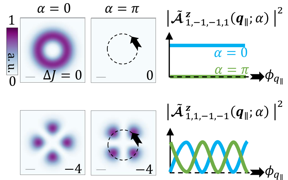
Longitudinal intensity
