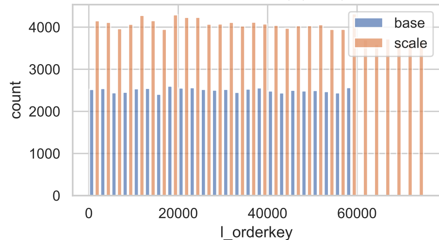
Lineitem order key (scale)
