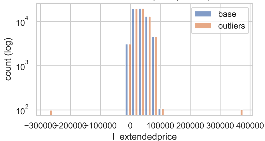
Lineitem extendedprice (outliers)
