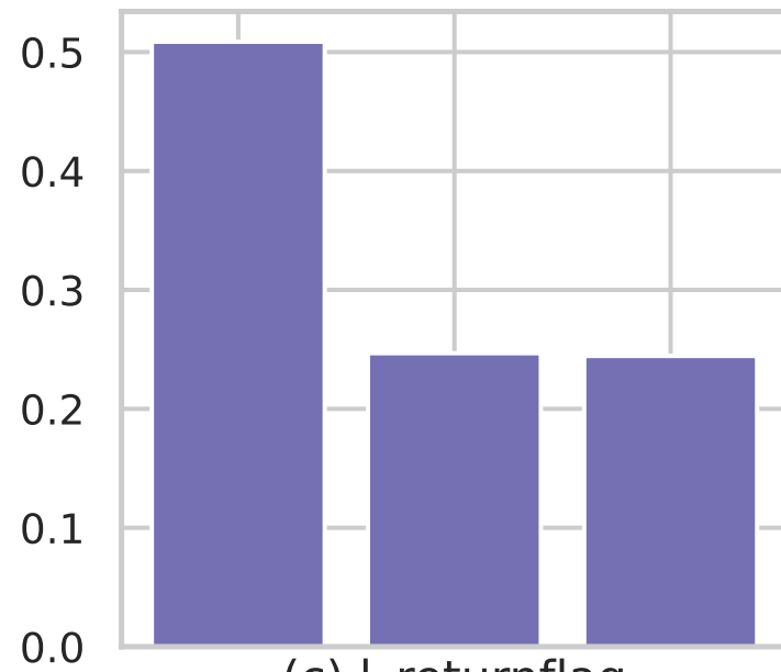
(c) l_returnflag
