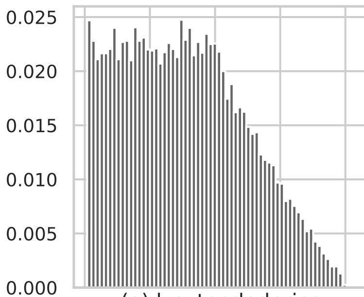
(e) l_extendedprice
