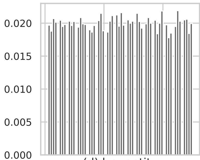
(d) l_quantity
