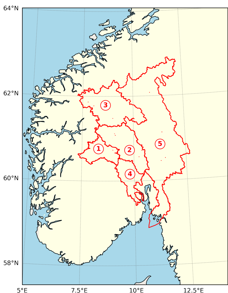
Summer (JJA)
