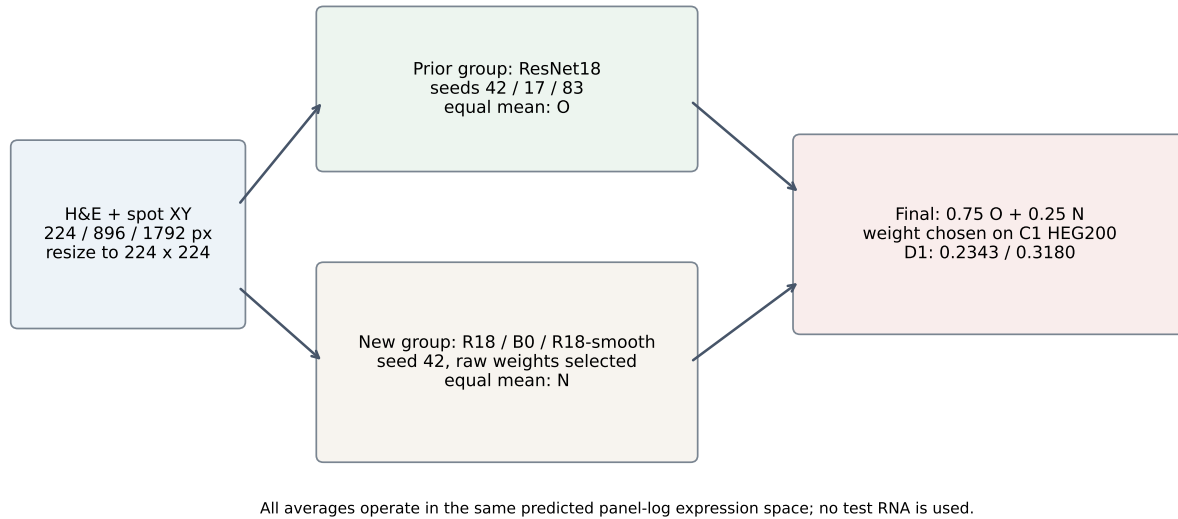
图 1: 最终集成的信息流。测试阶段只输入图像、坐标及固定面板元数据；C1 上选择的权重在 D1 推理时冻结。
