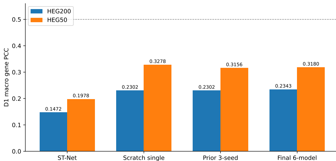
图 2: 固定面板宏平均 PCC。全随机单模型 HEG50 为 0.3278，高于最终集成的 0.3180；因此不能声称集成全面优于所有单模型。选择规则始终是 C1 HEG200，而不是 D1 HEG50。
