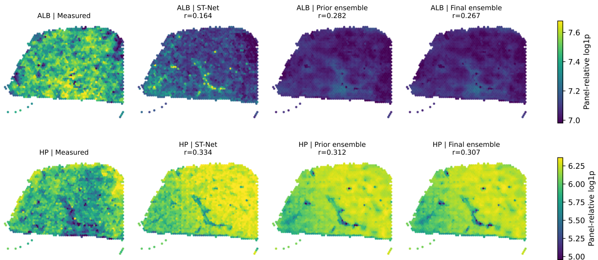
图 3: ALB 与 HP 的空间预测。沿用前轮已展示的基因作为示例，不据本轮测试 PCC 选择。每个基因的所有方法共用真值 1%–99% 分位色标，范围外颜色截断；PCC 仍使用完整未截断数值。个别示例不替代固定面板统计。
