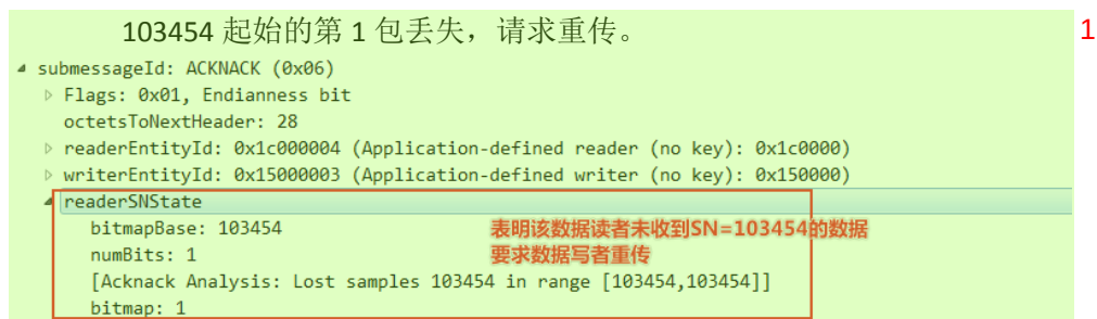
图 55 ACKNACK 子消息“NACK”
