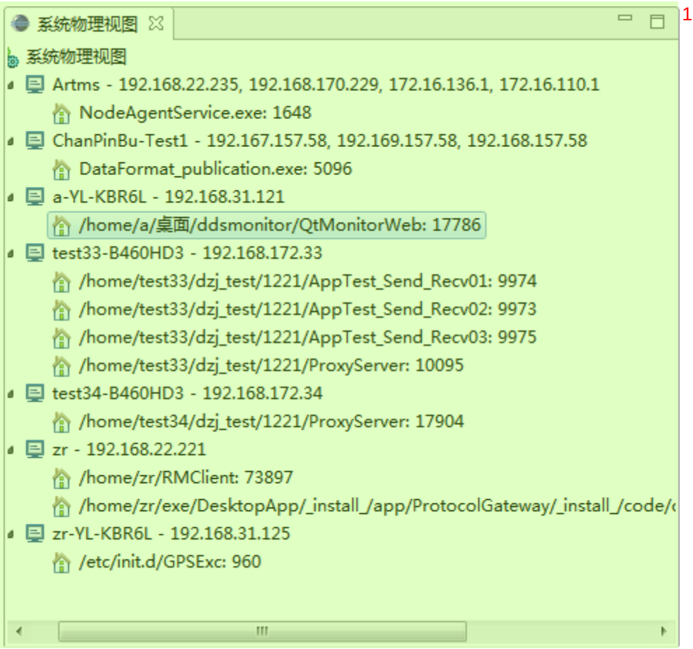
图 28 系统物理视图
