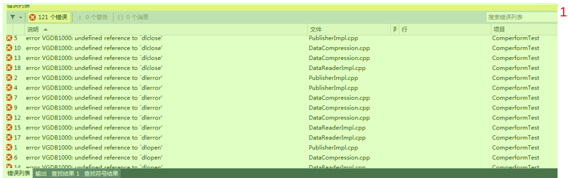
图 35 缺失 dl 库报错图
