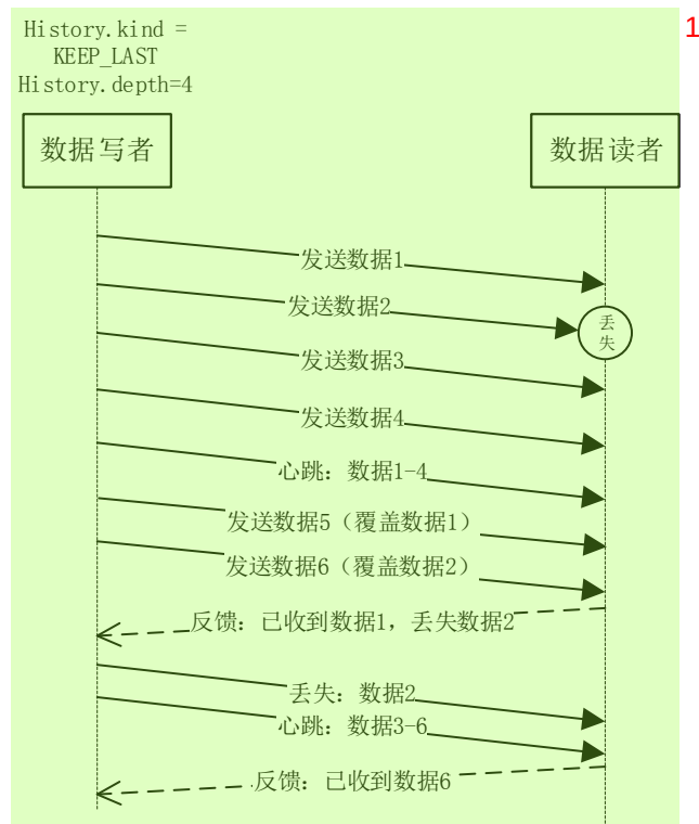
图 4 可靠模式下的数据覆盖 2
