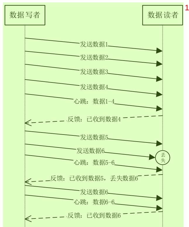
图 3 可靠模式通信 2
