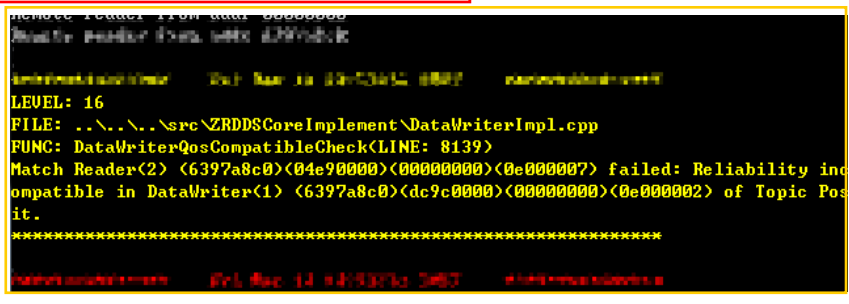
图 49 Qos 不匹配打印
