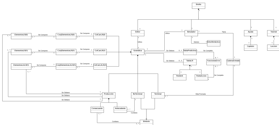
Figura 9.1: Diagrama de clases de SimAS 3.0
