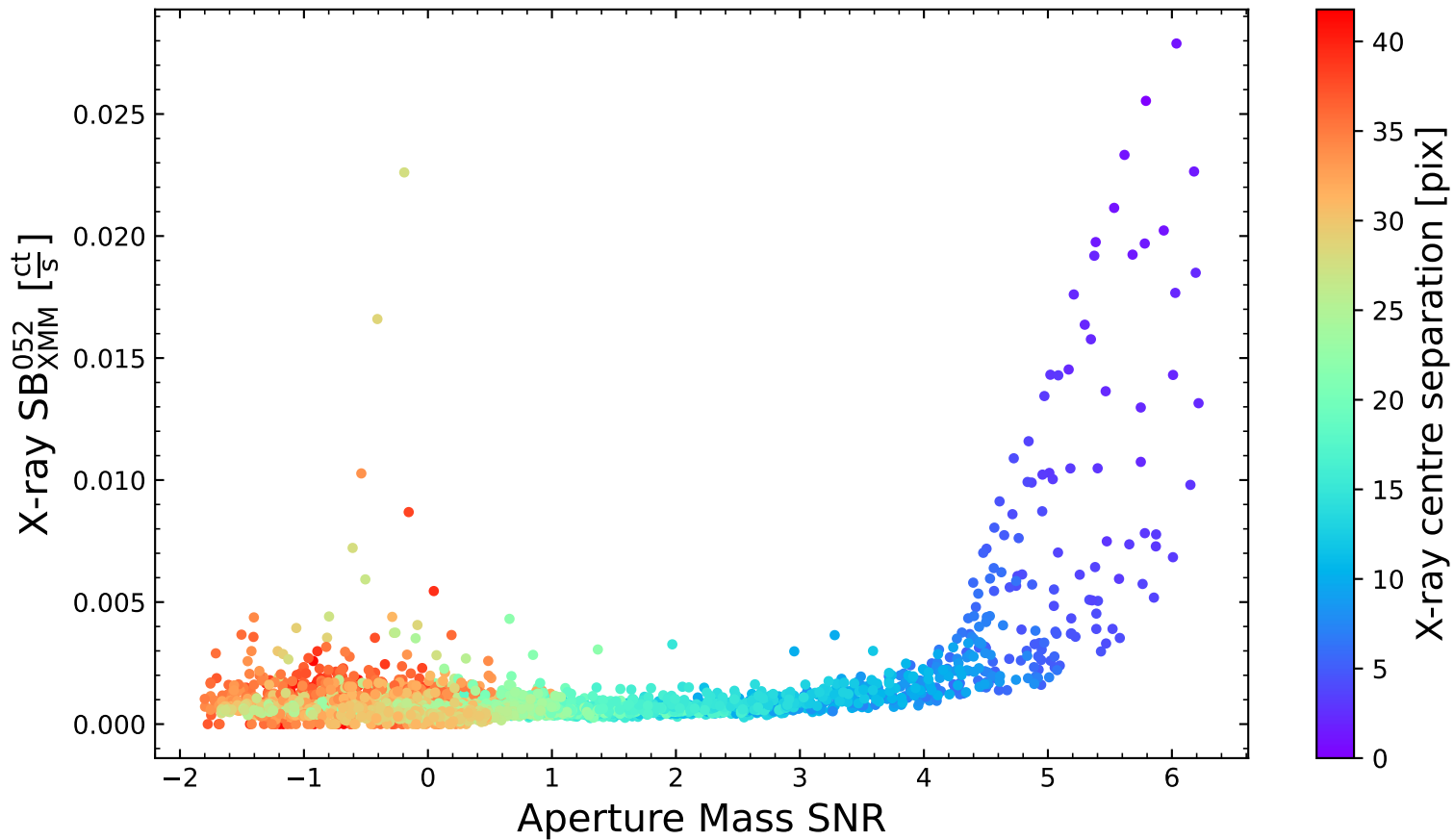
LoVoCCS-61
