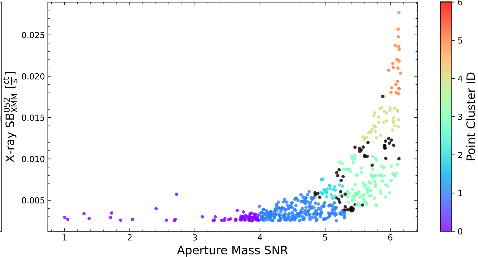
LoVoCCS-28
