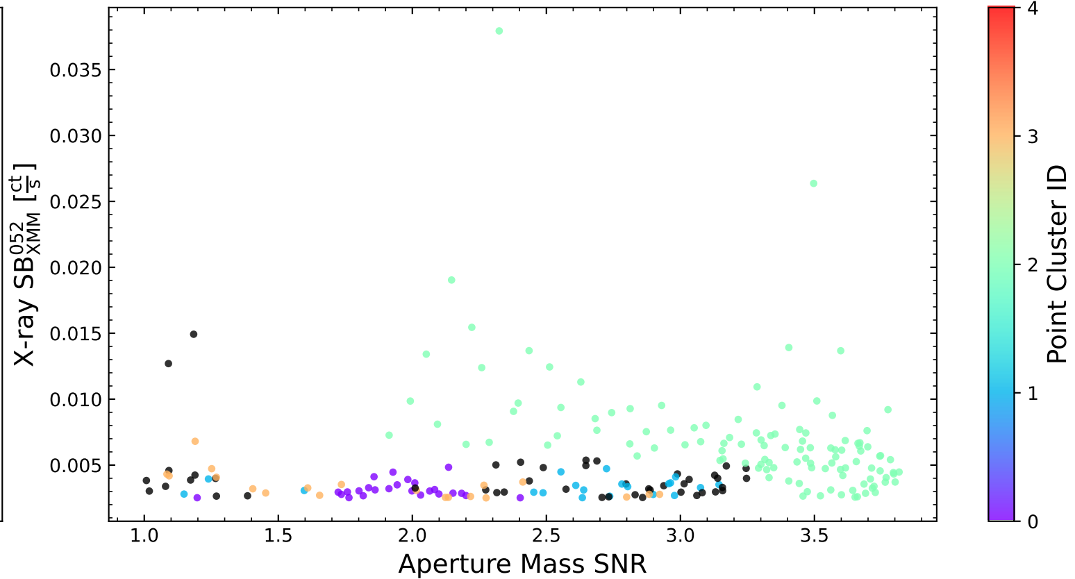
LoVoCCS-46
