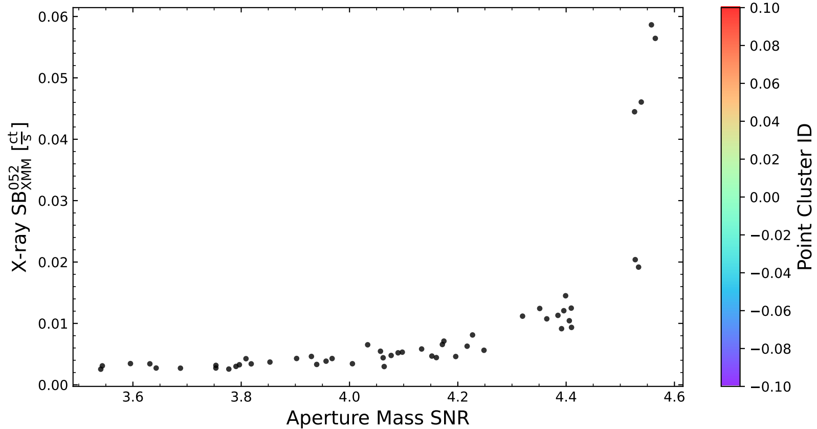
LoVoCCS-49
