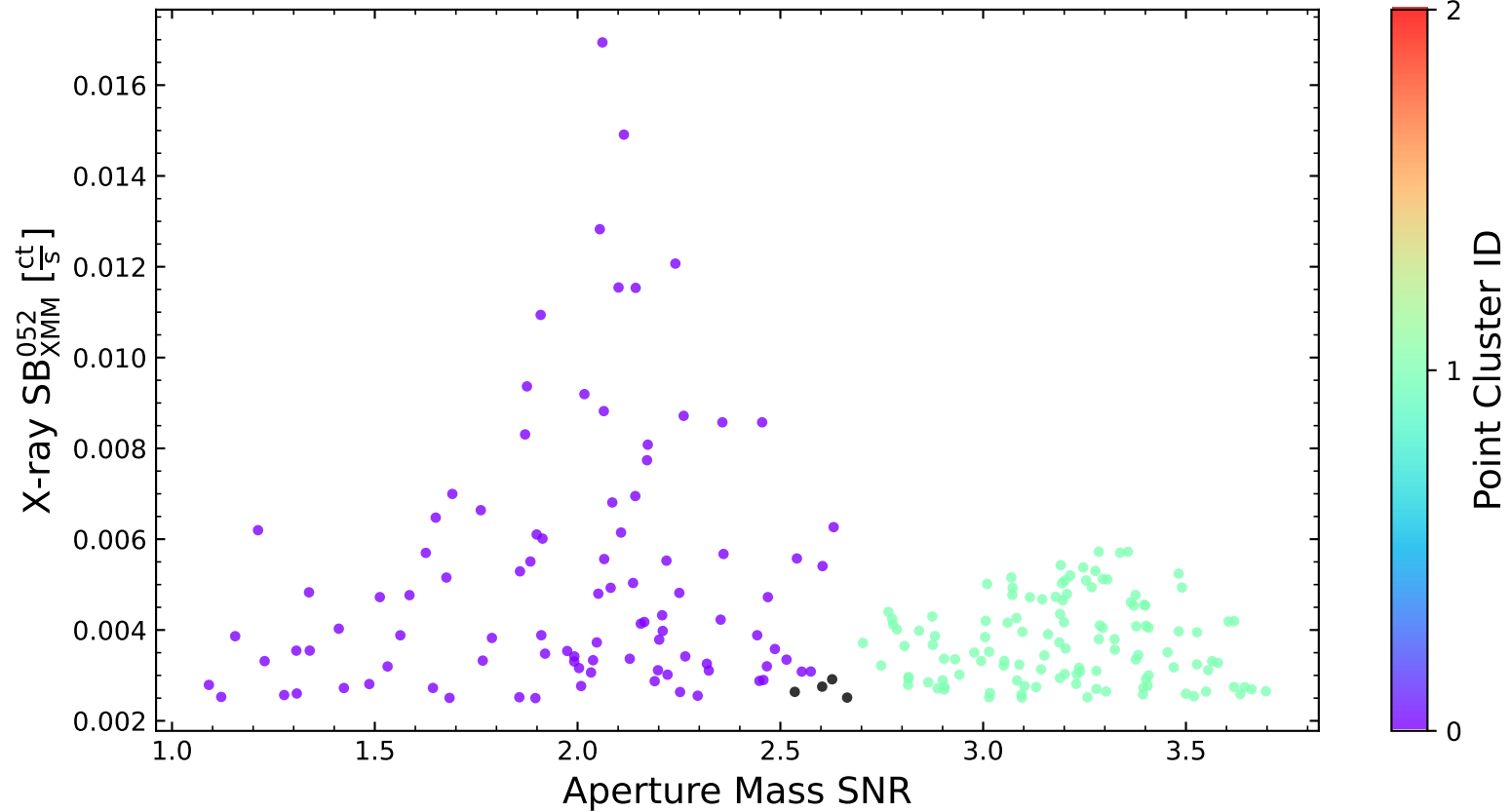
LoVoCCS-60
