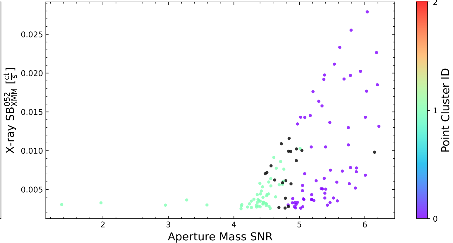
LoVoCCS-61
