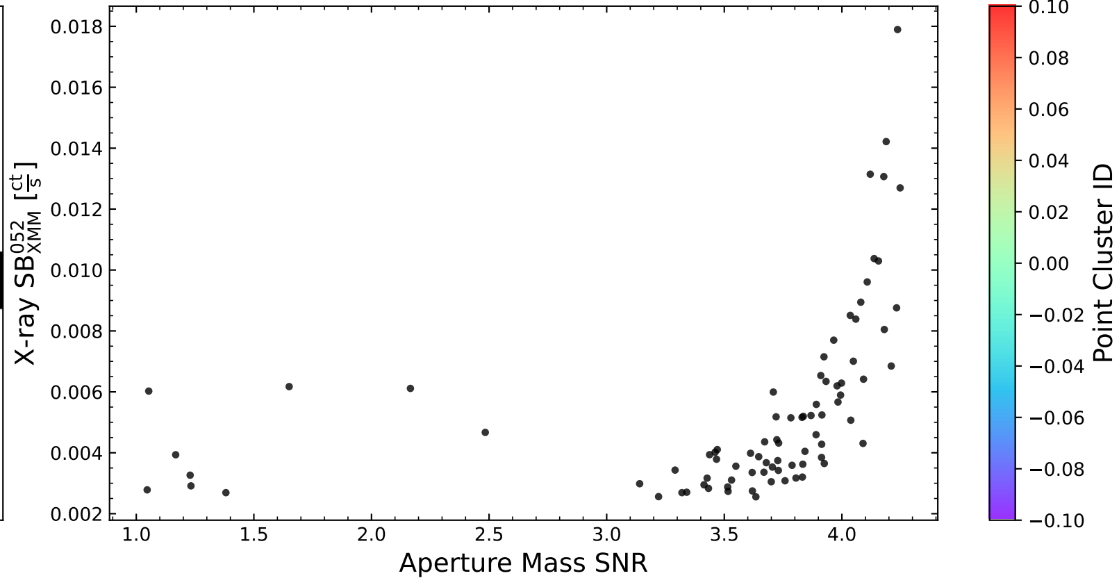
LoVoCCS-74
