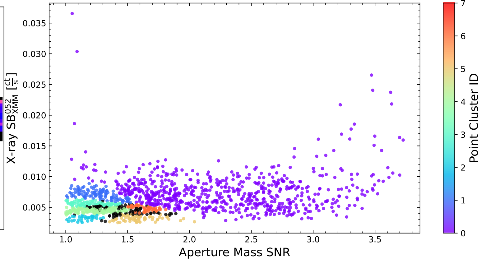
LoVoCCS-94
