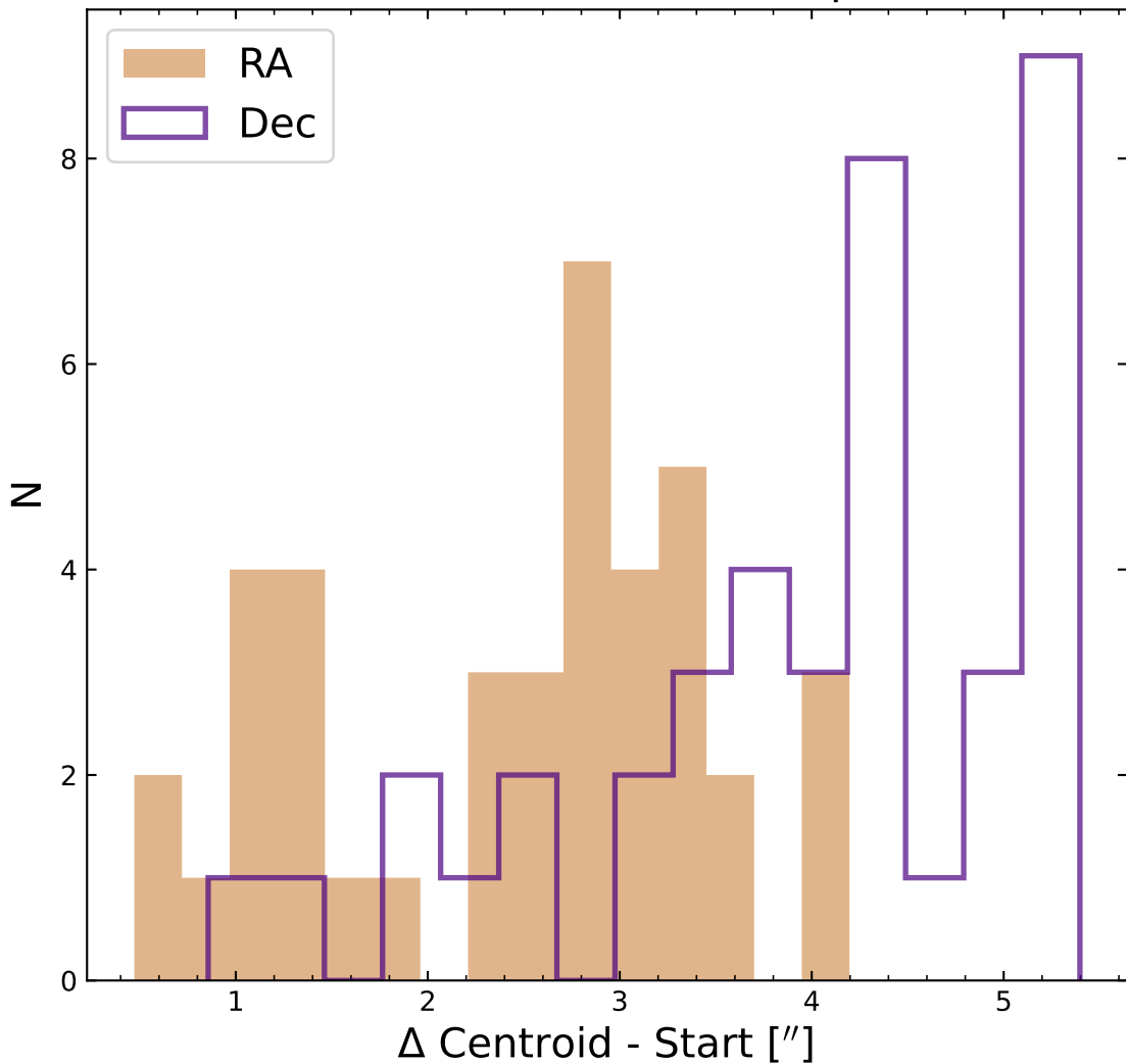
LoVoCCS-89 (100-500 kpc)
