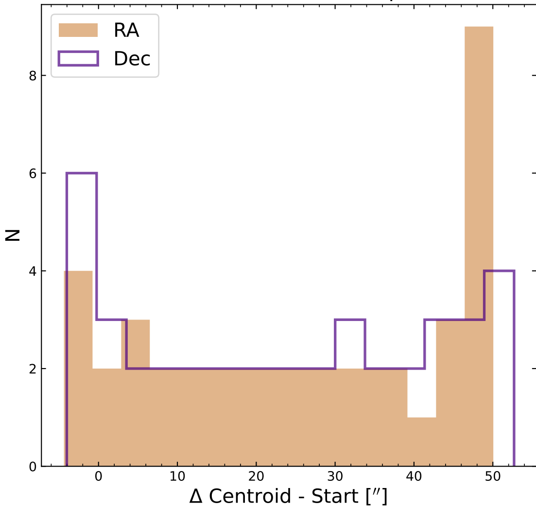
LoVoCCS-9 (100-500 kpc)
