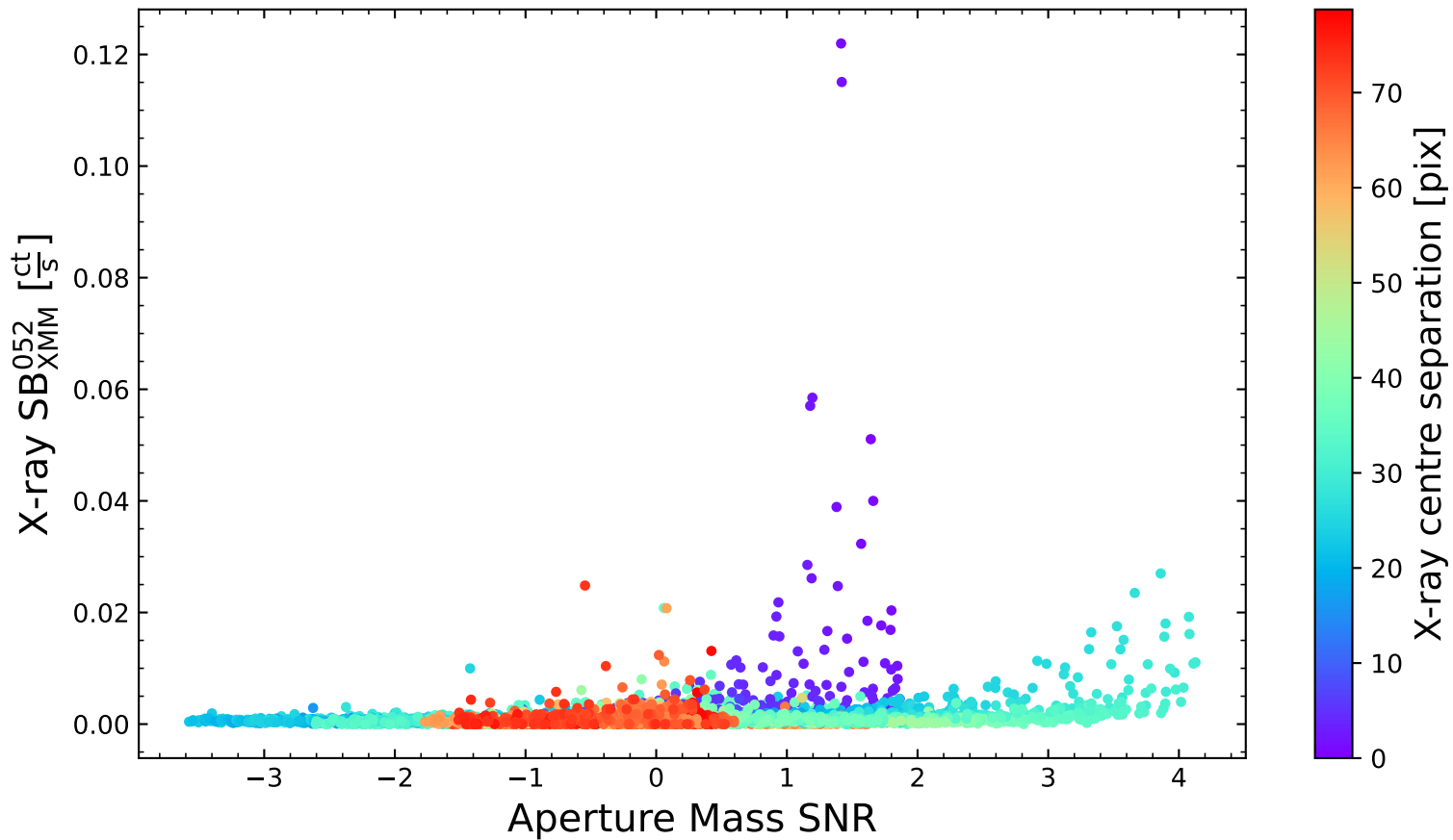
LoVoCCS-76
