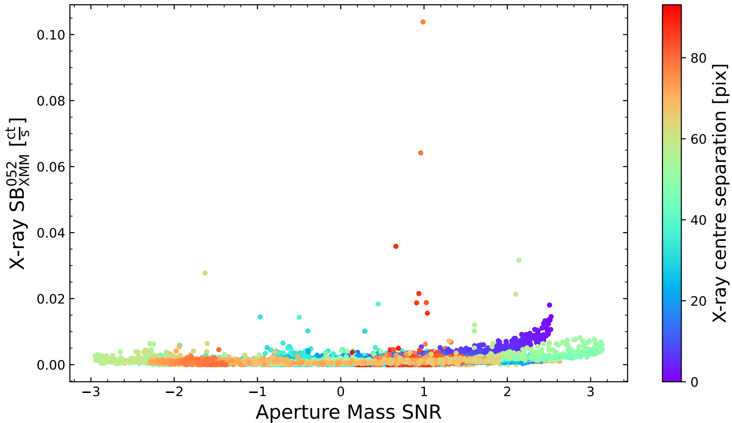
LoVoCCS-99
