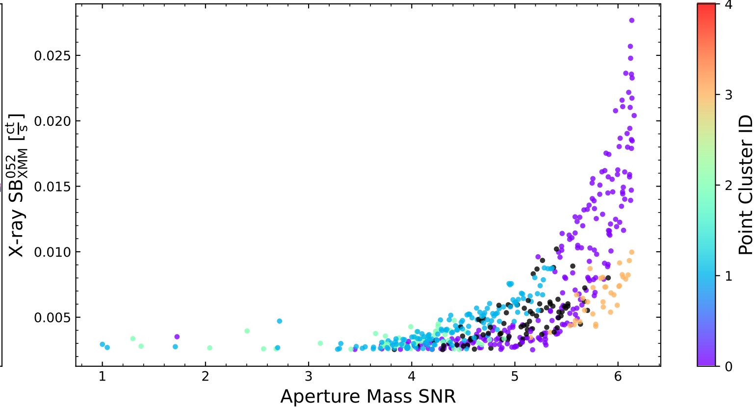
LoVoCCS-28
