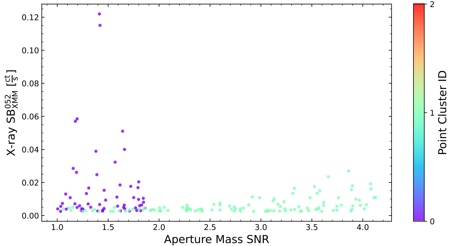
LoVoCCS-76
