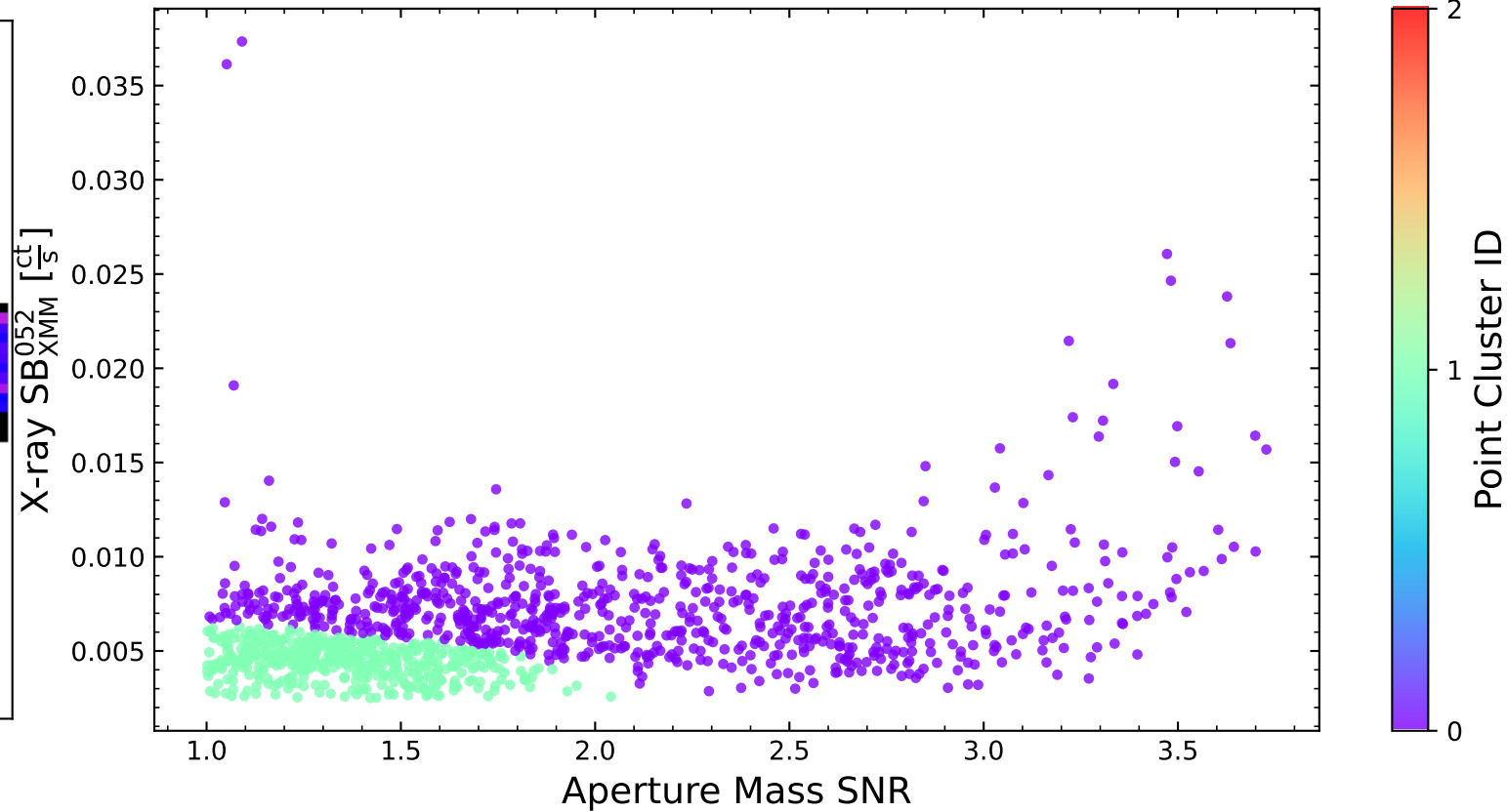
LoVoCCS-94
