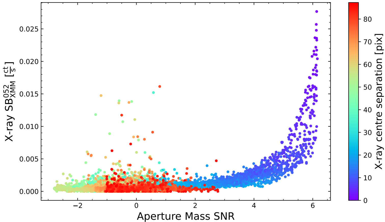
LoVoCCS-28
