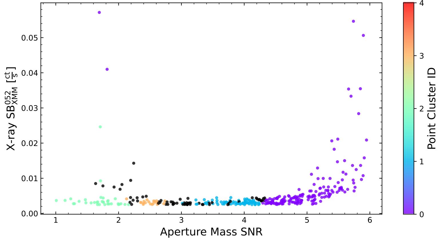
LoVoCCS-66
